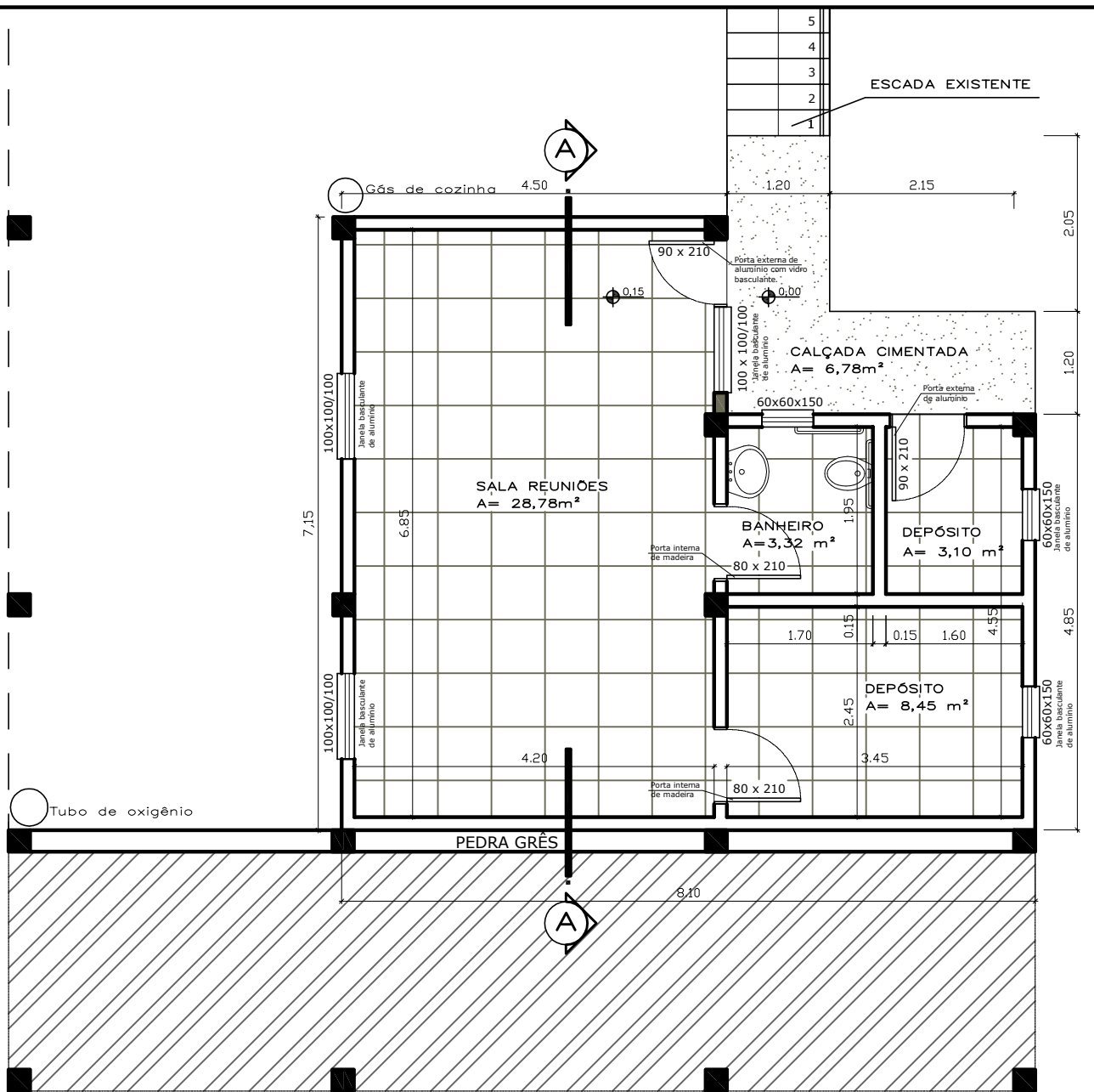
PLANTA BAIXA - Pavimento subsolo
