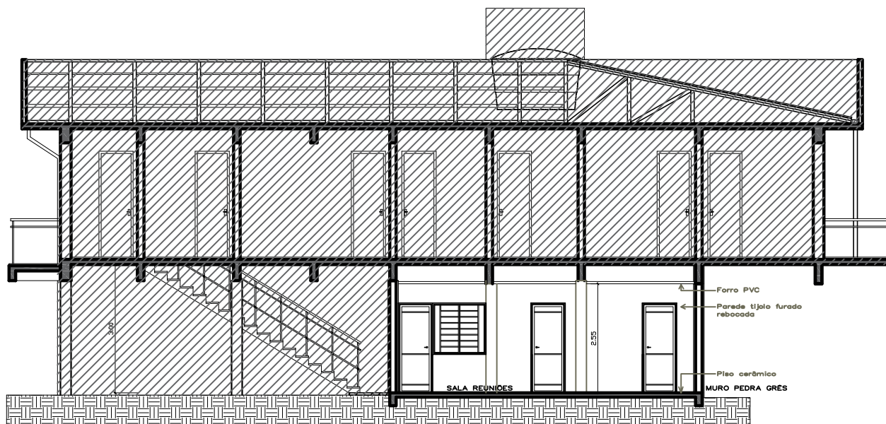
CORTE AA
