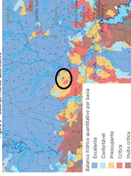
Figura 9 – Balanço Hídrico Quantitativo
