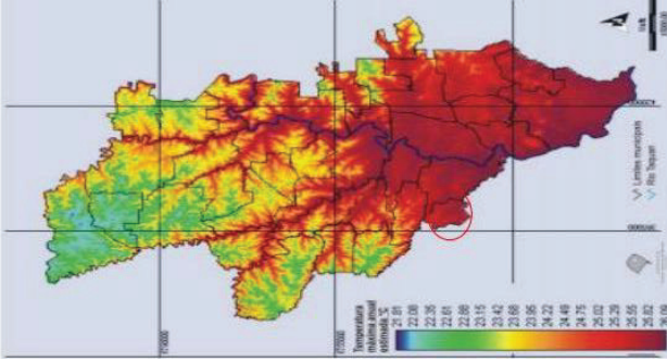
Figura 7 – Estimativa das temperaturas médias máximas anuais para o Vale do Taquari - RS
