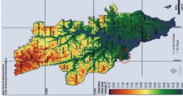
Figura 6 – Estimativa das temperaturas médias anuais para o Vale do Taquari - RS
