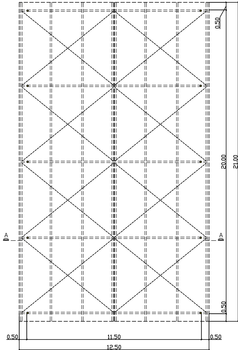
PLANTA DE PILARES COM PROJEÇÃO DA COBERTURA
